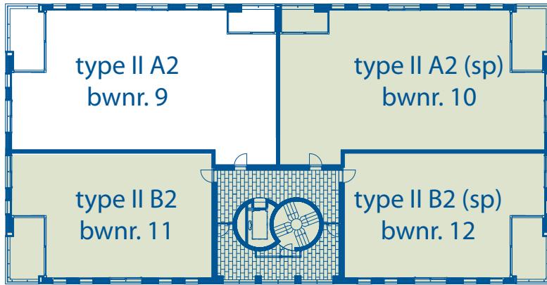
VILLA TYPE II Tweede Verdieping
