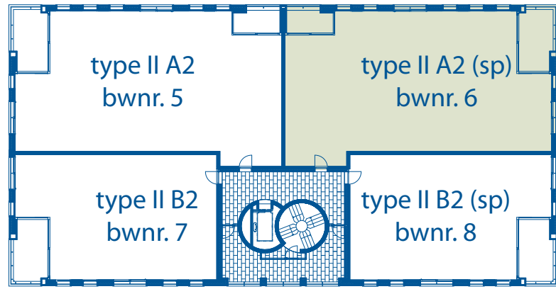
VILLA TYPE II Eerste Verdieping
